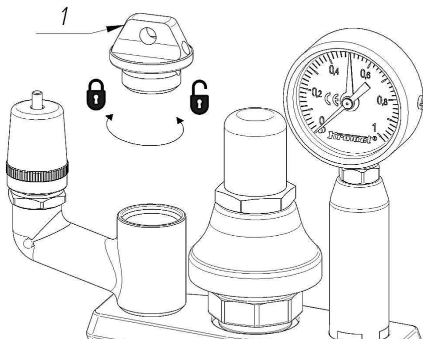
rys 9. Schemat usytuowania korka i króćca wlewowego
