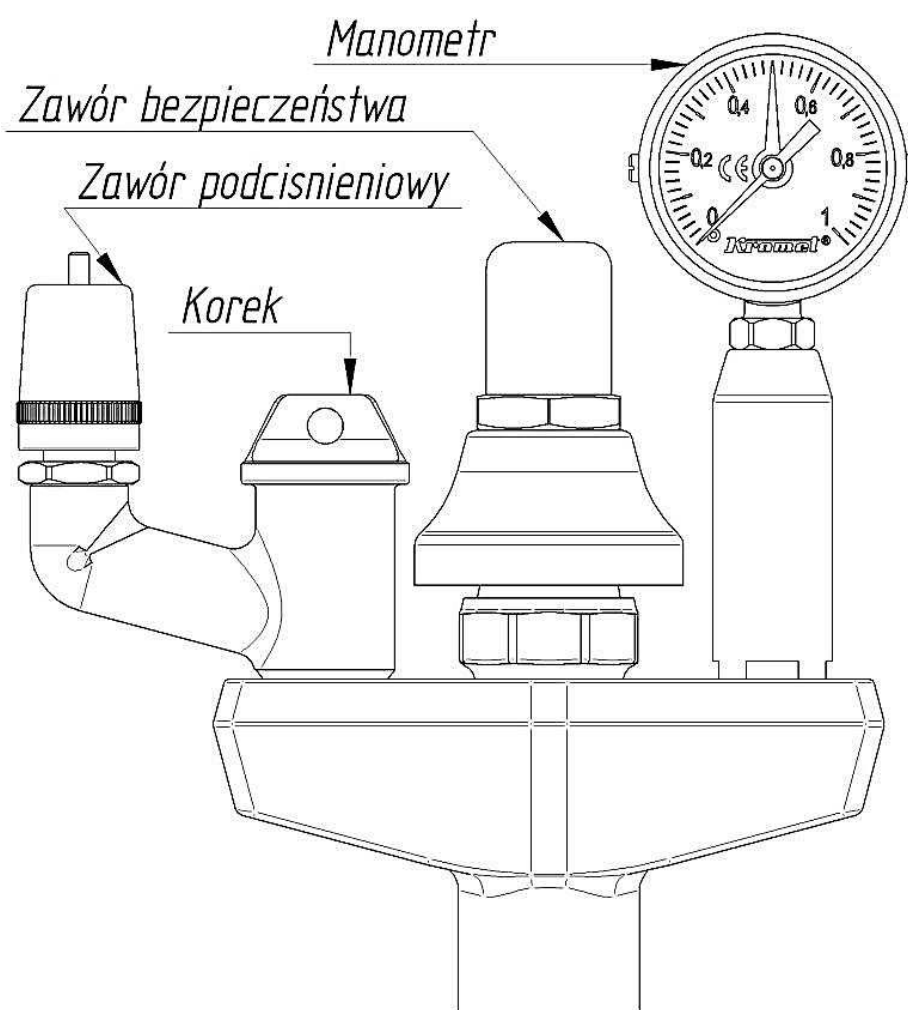
rys 3. Opis zespołu zabezpieczającego
